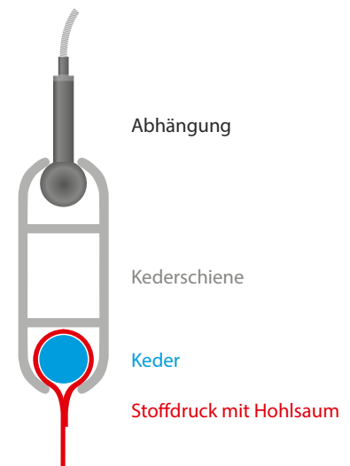
Schematische Darstellung: Abhängung per Keder und verstellbarem Nutenstein
